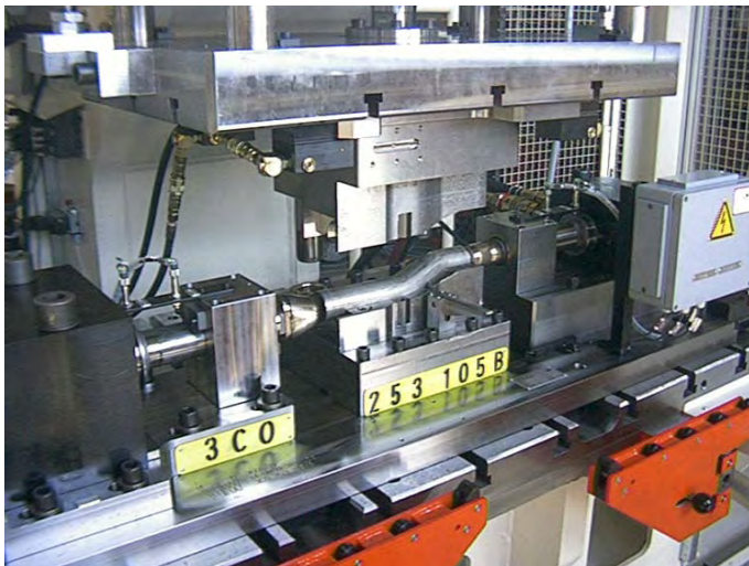
Formwerkzeug, eingebaut in Universal-Formvorrichtung
