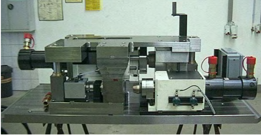
Formwerkzeug, im ausgebauten Zustand
